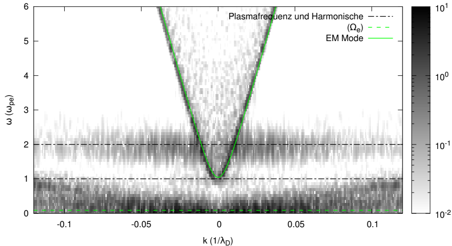
B_z , 27 grad gegen die Beam-Richtung (transversal)
